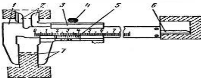
Рис. 1. Штангенциркуль:
