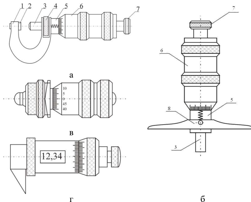
Рис. 8. Микрометрические инструменты:
