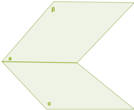
Рис. 3. Двугранный угол.
