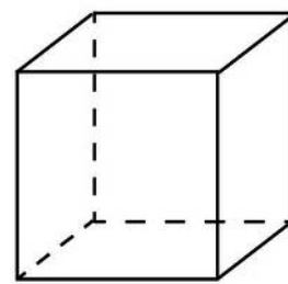
Правильный гексаэдр
