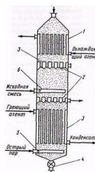
Рис. 3 Адсорбер с движущимся слоем
