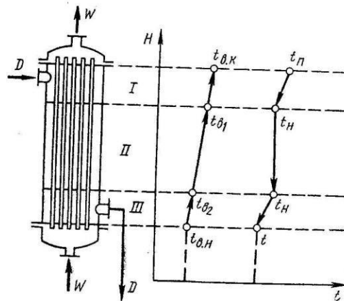
Рис. 1 Кожухотрубный конденсатор
