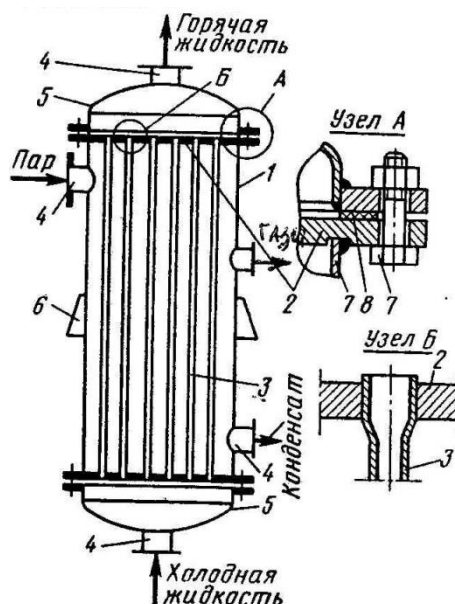
Рис. 1 Схема вертикального однокотлового кожухотрубчатого теплообменника с неподвижными трубчатыми решетками (а) и размещение труб в трубчатой решетке (б):
