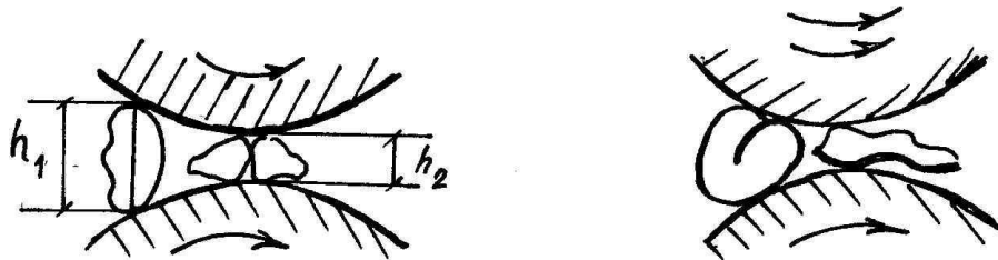
Рис.3 Схем деформации зерна: а – сжатие; б – сдвиг.
