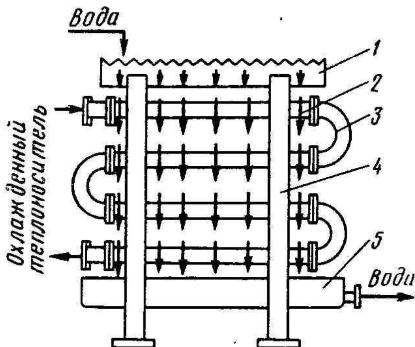
Рис.3 Оросительный теплообменник:
