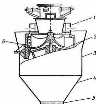
Рис. 8 Рамная центробежная свеклорезка:
