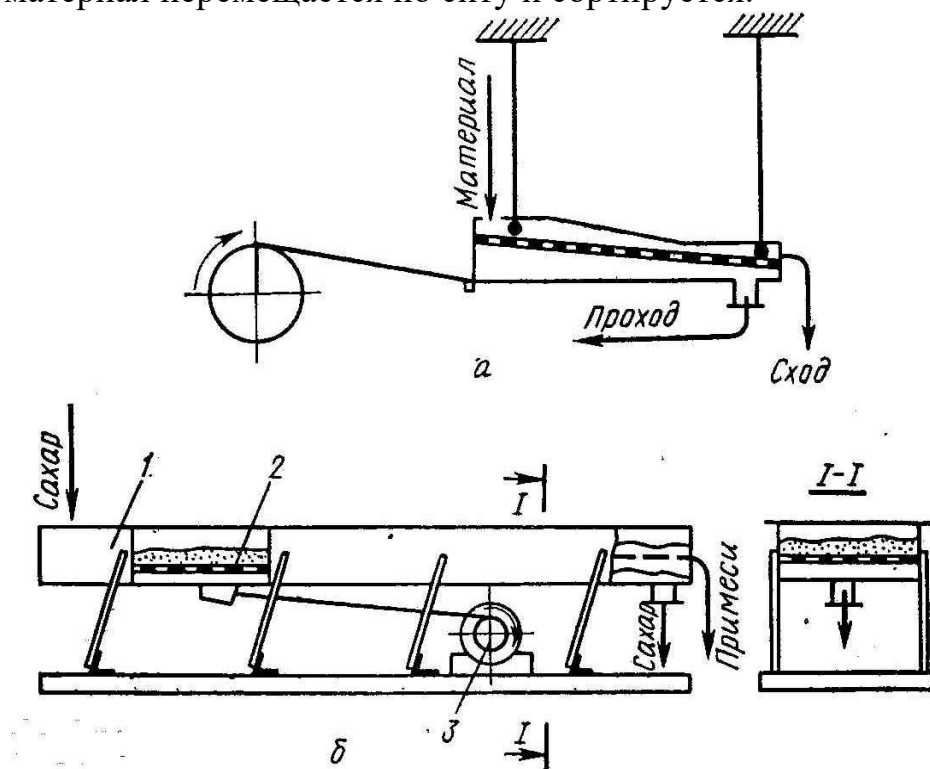
Рис.1 Схемасортировочныхситовыхмашин: а–качающегося сита;б – трясуна.
