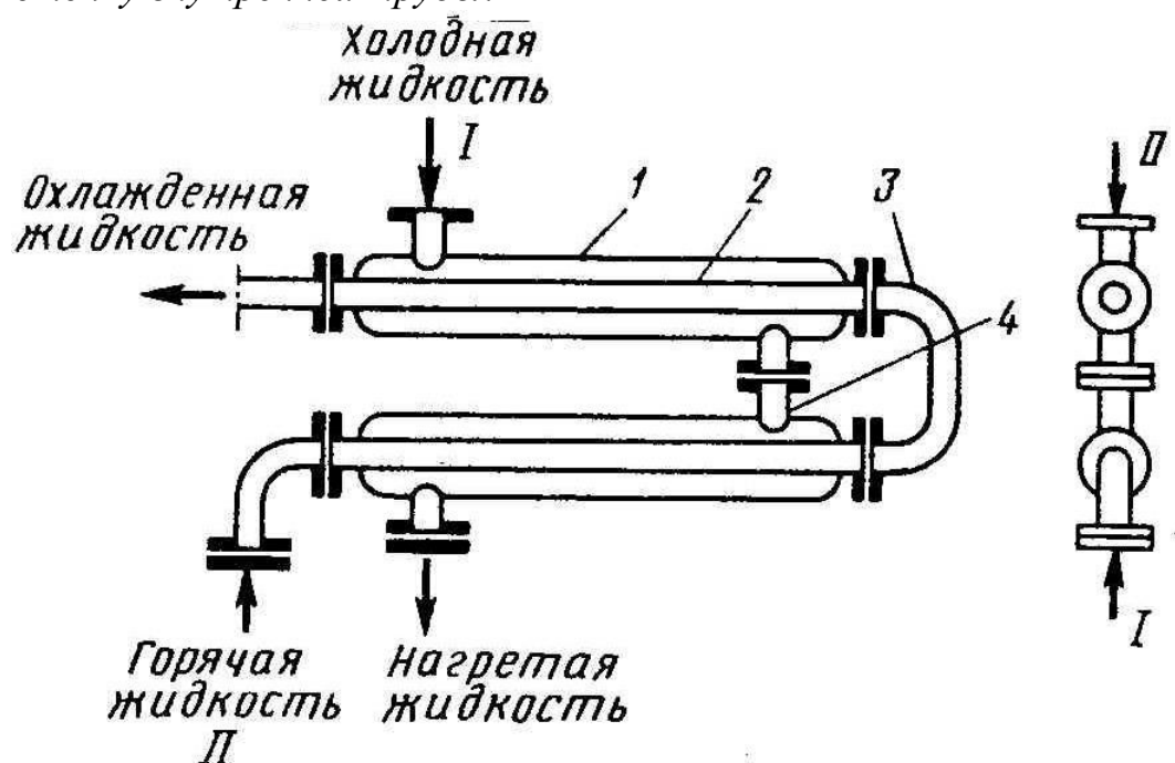
Рис. 2 Теплообменник типа «труба в трубе»: 1 – наружная труба; 2 – внутренняя труба; 3 – колено; 4 – патрубок; I, II – теплоносители
