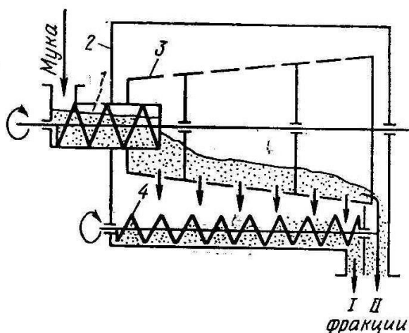
Рис. 2 Схема бурата:
