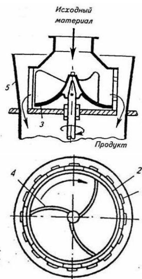
Рис. 9 Центробежная резка для измельчения свеклы:
