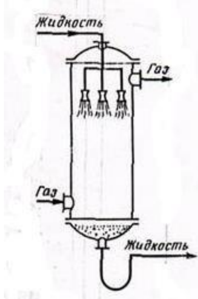
Рис. 7 Распыливающий абсорбер
