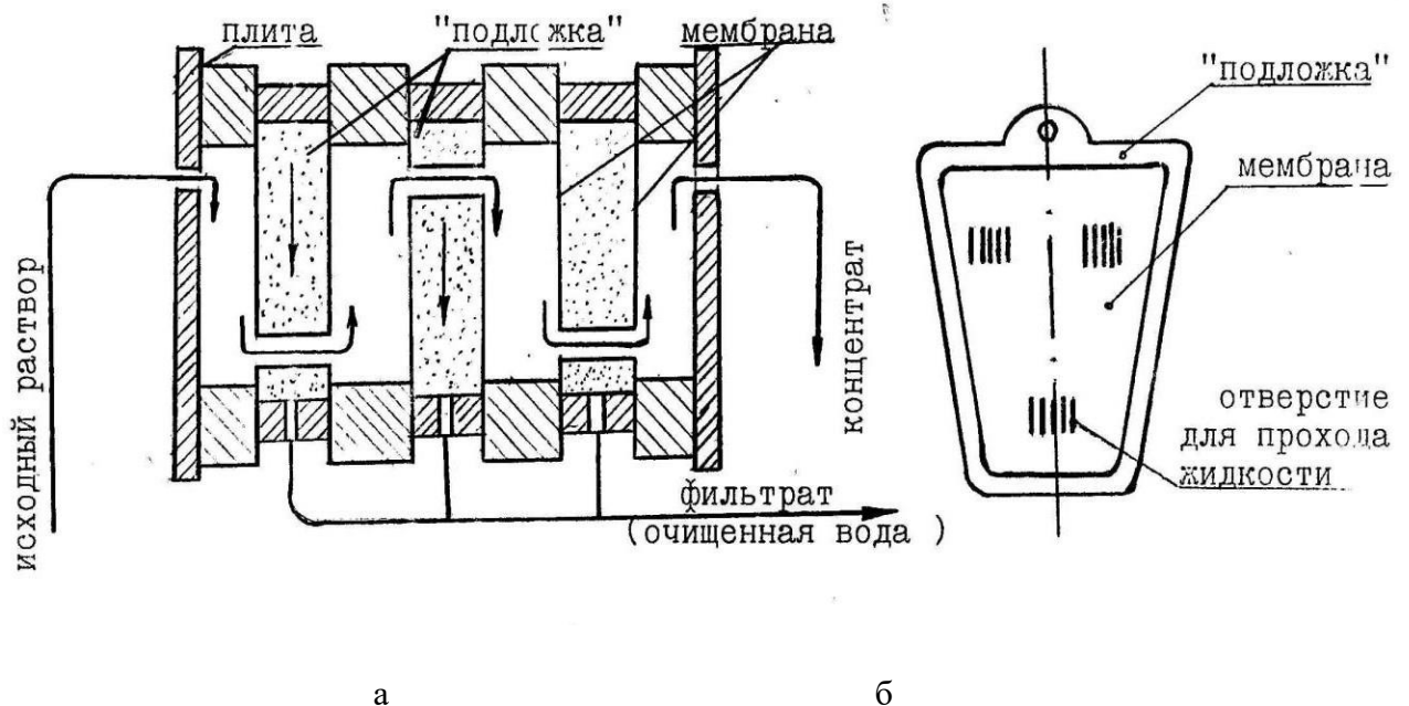
Рис. 1 Мембранный фильтр-пресс (а) и «подложка» (б)
