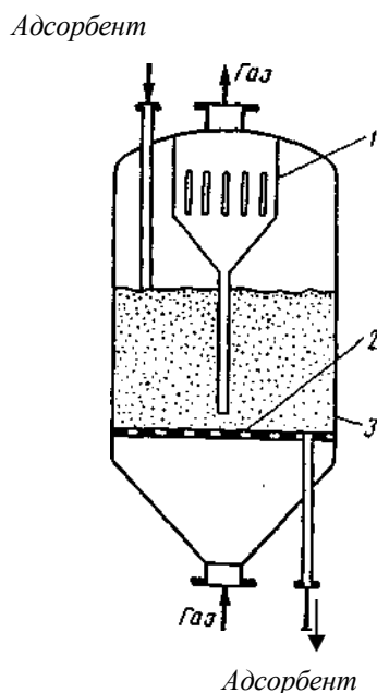
Рис. 4 Одноступенчатый адсорбер непрерывного действия с псевдооживленным слоем:
