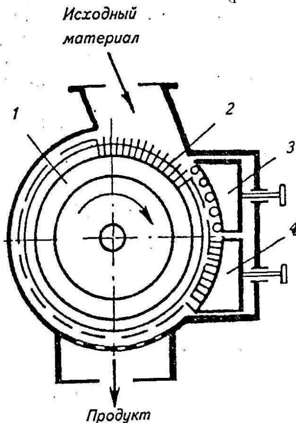
Рис.7Схемакартофелетерки
