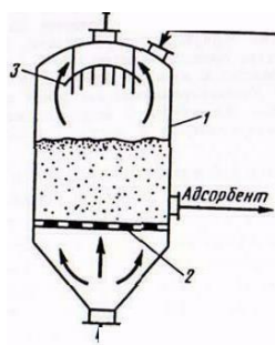
Рис.2 Одноступенчатый адсорбер непрерывного действия с псевдоожиженным слоем
