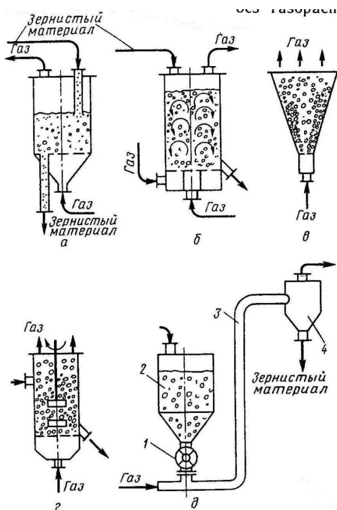
Рис.1 Схемы аппаратов псевдоожиженным слоем:
