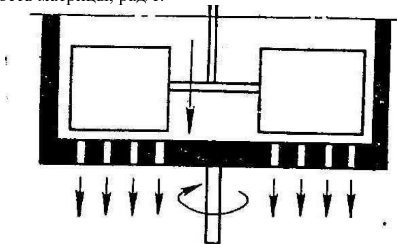
Рис. V—2. Схема ротационного пресса
